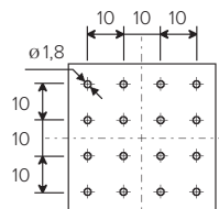
RDMM (per c.s.) Piano di foratura (vista lato saldatura)
