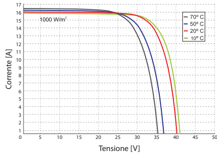
Curva I-V a varie temperature delle celle
